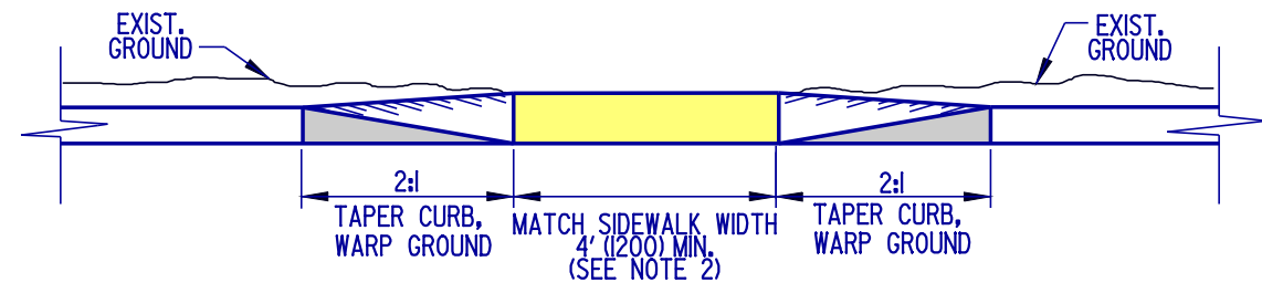
ELEVATION A-A
