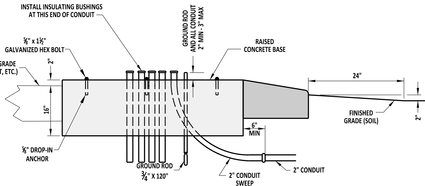
SECTION A-A
